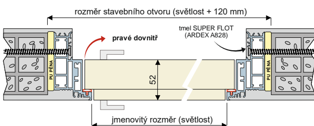
FORTIUS 52 zárubeň pro zdivo, otevírání dovnitř – reverzní
