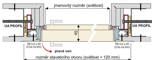
DURUS 45 zárubeň pro SDK, jednoduché opláštění, otevírání ven
