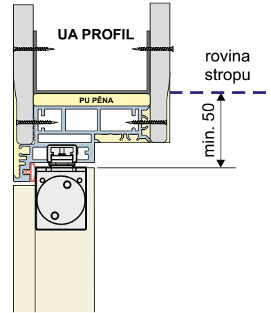
Otevírání DOVNITŘ
