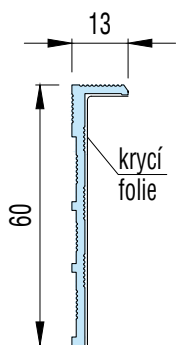
soklová lišta LINUS 13
