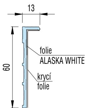
soklová lišta LINUS 13
