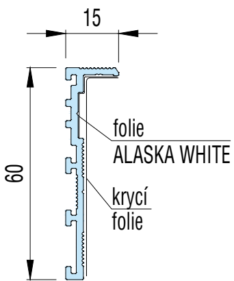
soklová lišta LINUS 15 pro LED
