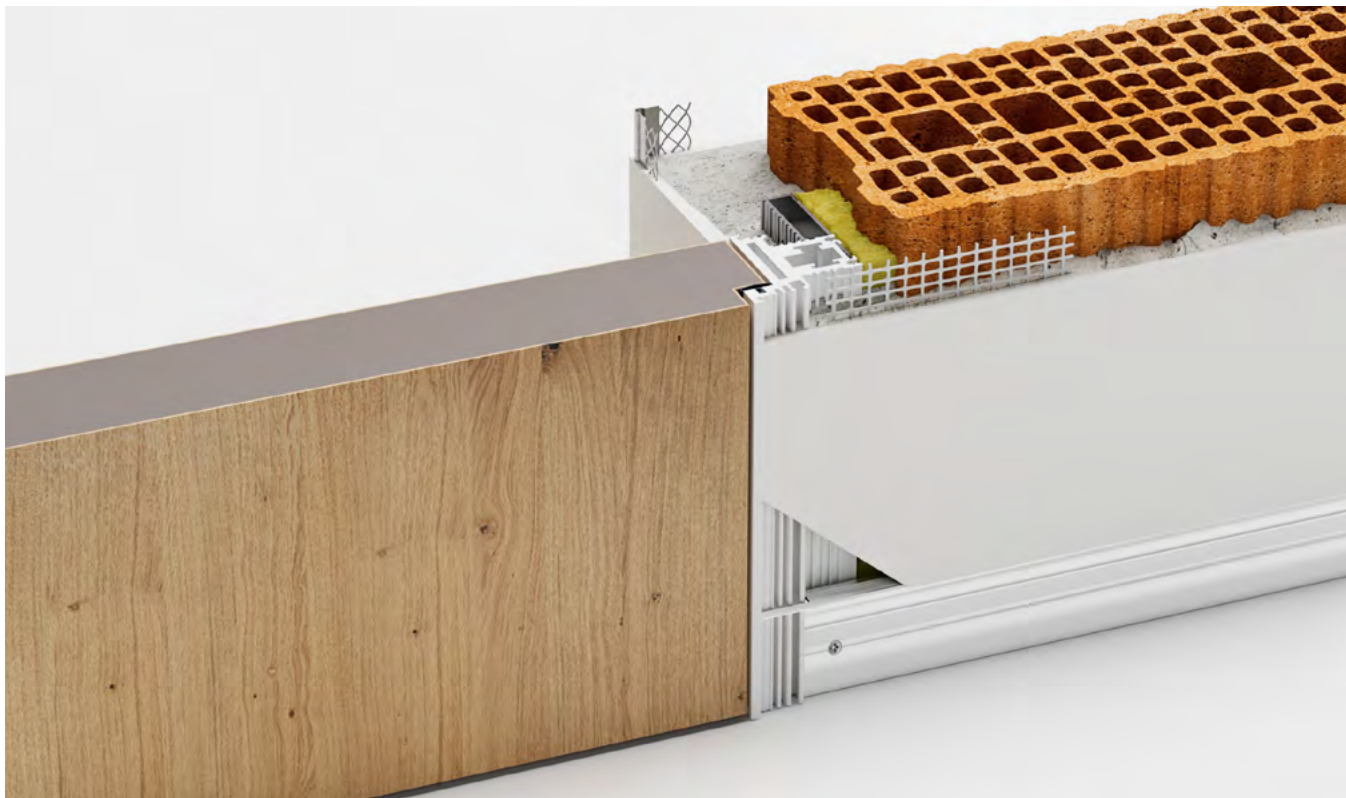
FORTIUS 52 - otevírání dovnitř, líčující strana
