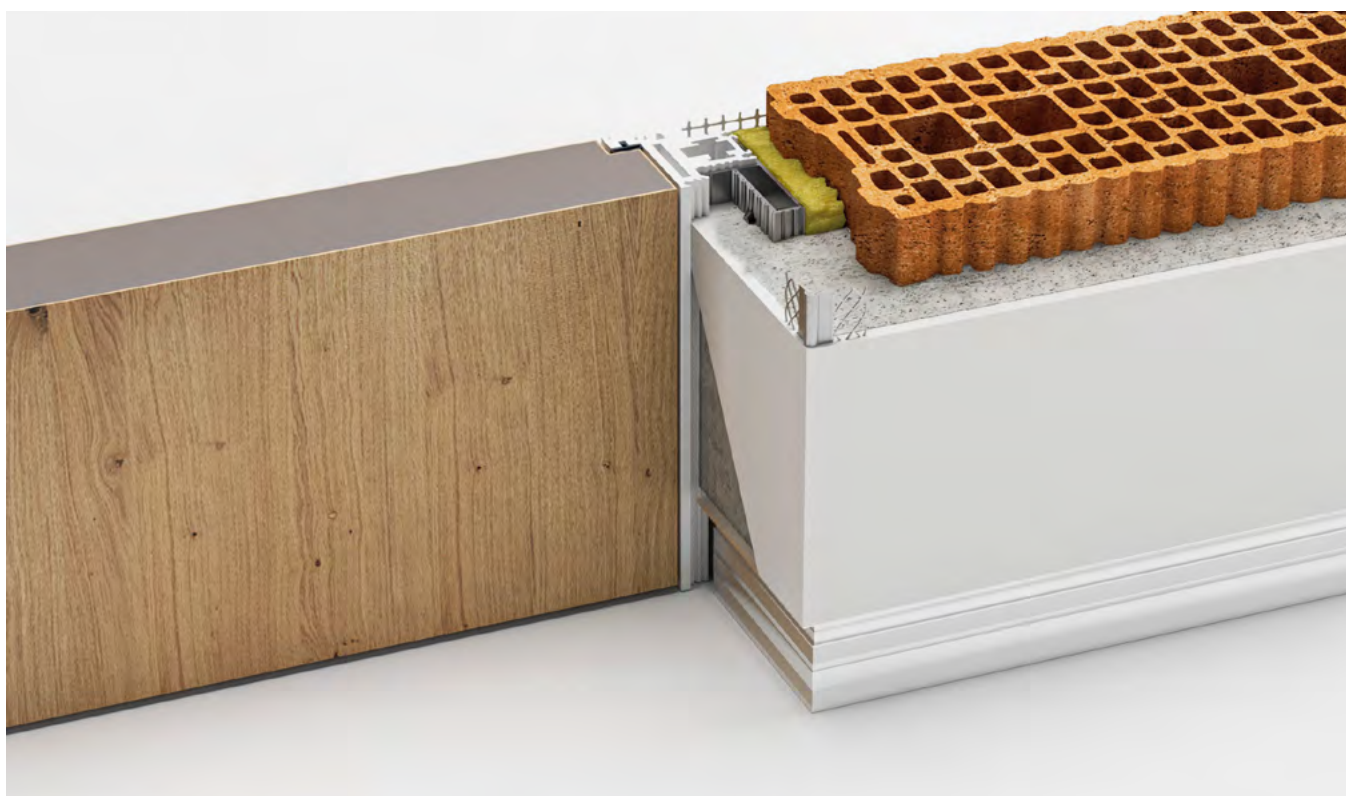
FORTIUS 52 - otevírání dovnitř, rubová strana
