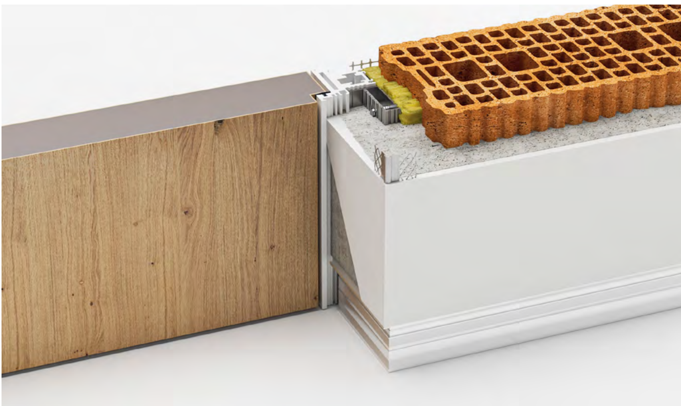
FORTIUS 52 - otevírání ven, rubová strana
