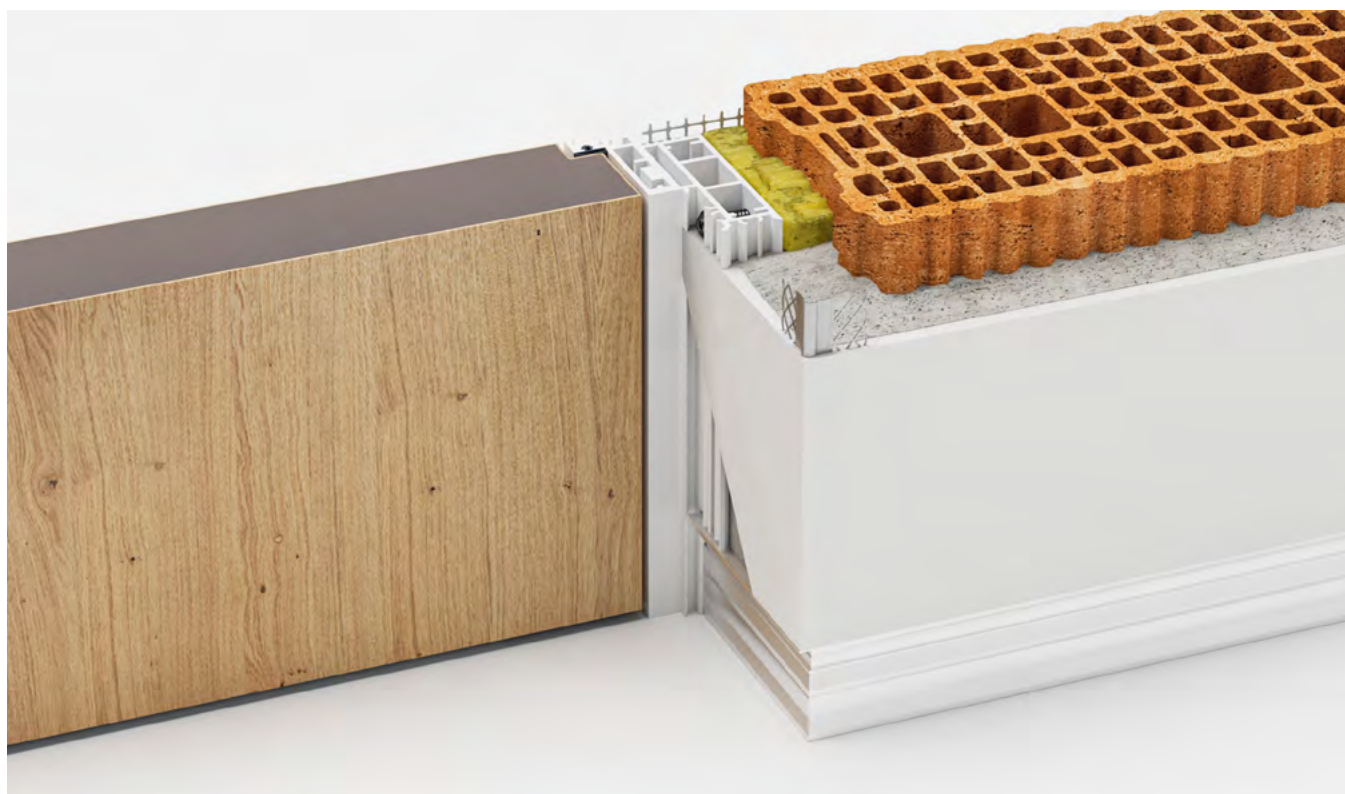
FORTIUS 52 XR NEW - otevírání dovnitř, rubová strana
