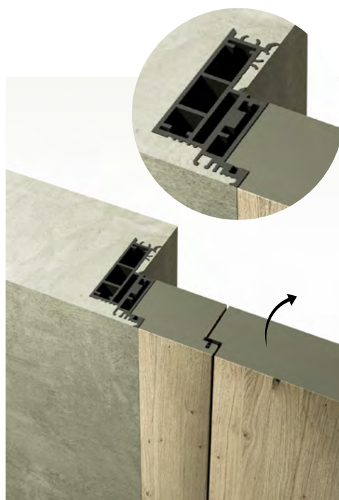
Fortius woody otevírání dovnitř
